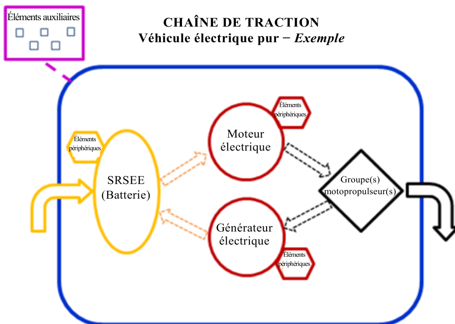
Figure 3 Véhicule électrique pur – VEP
