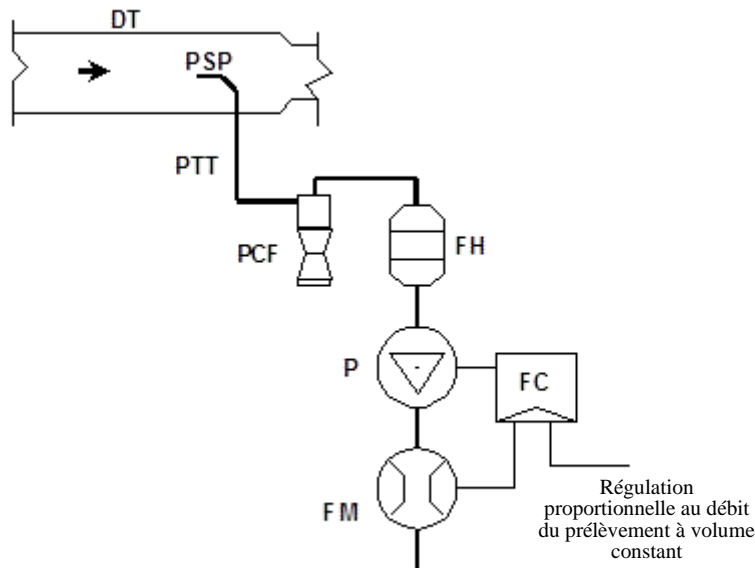
Figure B.2.-5 Système de prélèvement d'échantillons de particules
