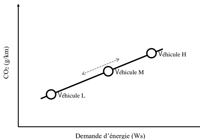
Figure A8/5 Limites pour la sélection du véhicule M
