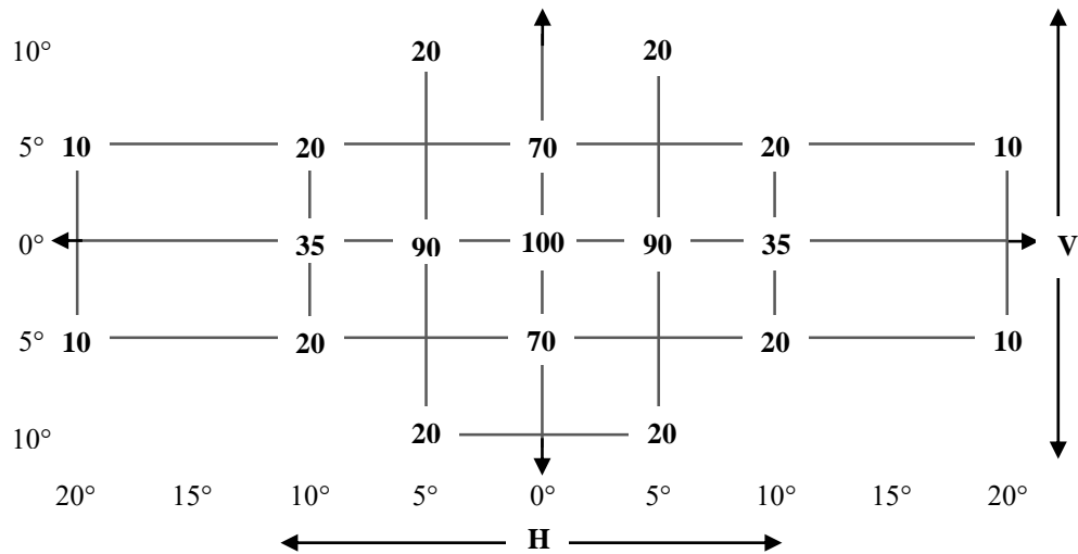
Стандартное распределение света передних и задних габаритных, стояночных, контурных огней, сигналов торможения и указателей поворота
