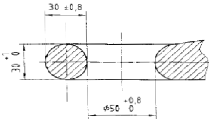
Figure 10 Dimensions des anneaux de timon toriques de la classe d50-1
