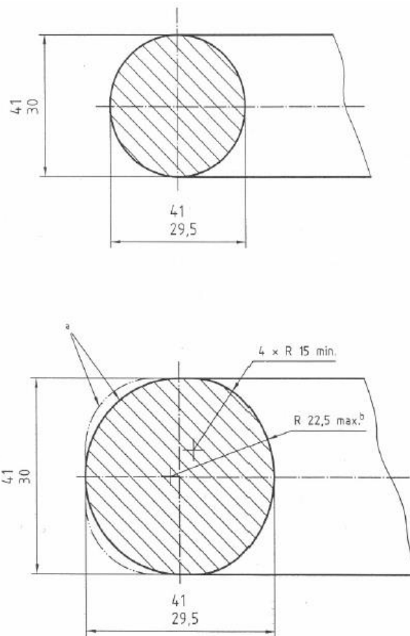
Figure 11 Dimensions des anneaux de timon toriques de la classe d50-2
