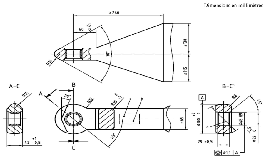
Figure 8 Dimensions principales des anneaux de timon de la classe d40-2
