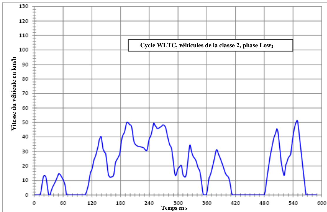
Figure A1/3 Cycle WLTC, véhicules de la classe 2, phase Low 2
