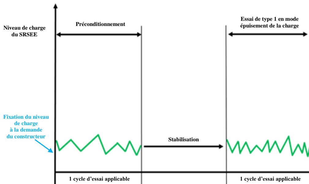
Figure A8.App1/5 VHE-NRE et VHPC-NRE, essai de maintien de la charge du type 1
