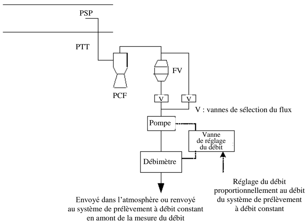
Figure A5/13 Système de prélèvement d'échantillons de particules à double dilution
