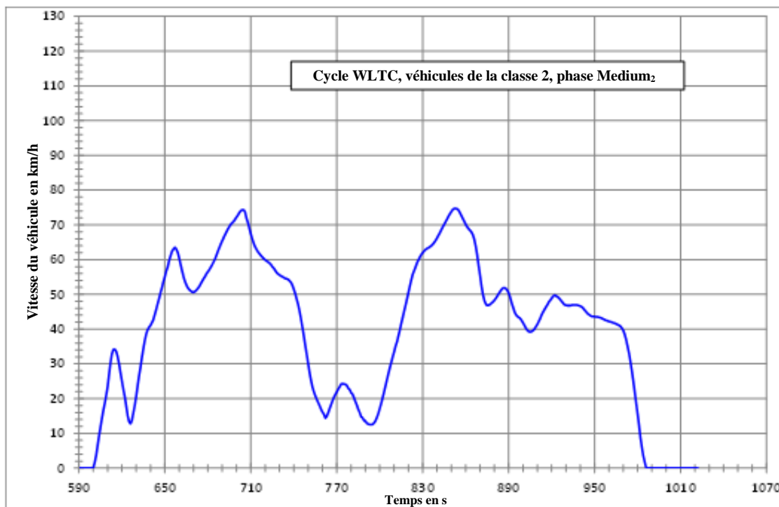
Figure A1/4 Cycle WLTC, véhicules de la classe 2, phase Medium 2
