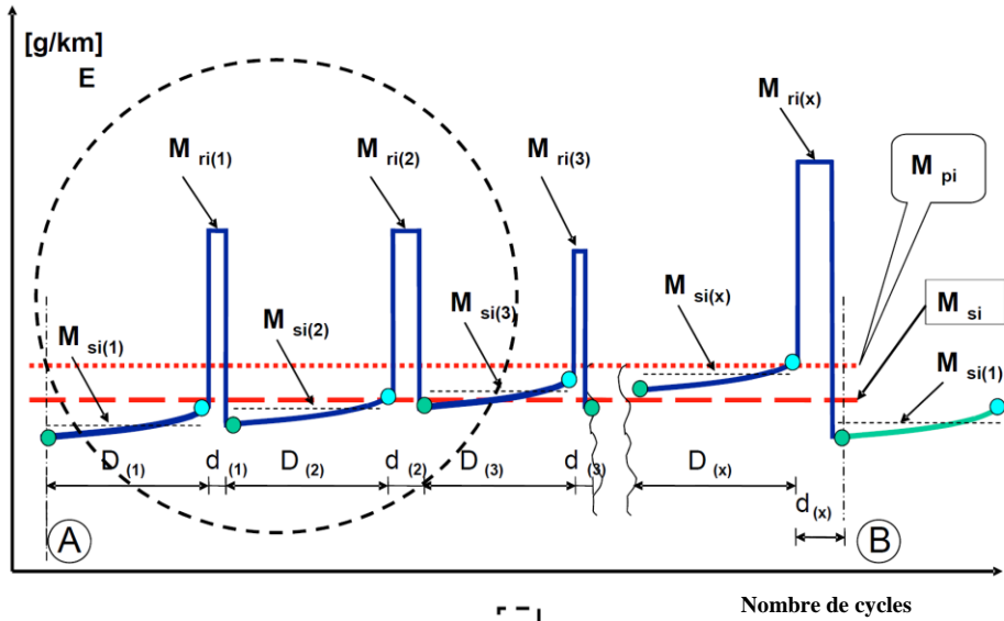
Figure A6.App1/2 Paramètres mesurés lors des essais d'émissions pendant et entre les cycles où se produit une régénération (il ne s'agit que d'un exemple)
