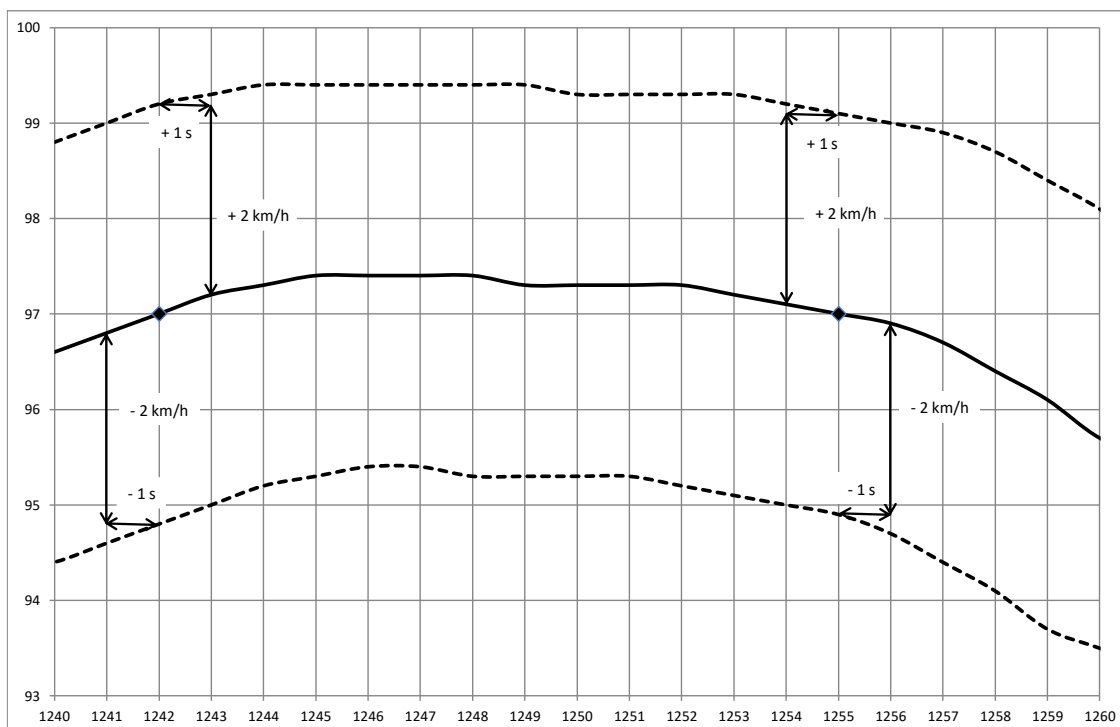
Figure A6/2 Tolérances par rapport à la courbe de vitesse
