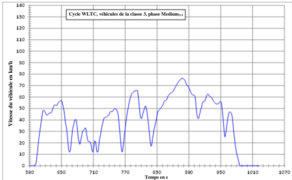
Cycle WLTC, véhicules de la classe 3, phase Medium 3,1
