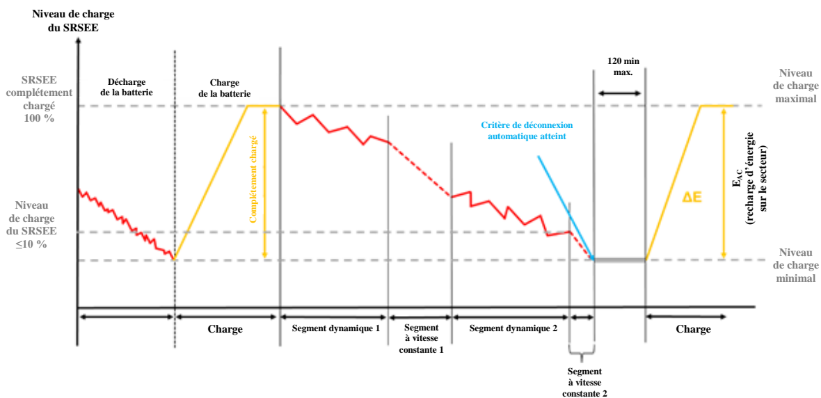
Figure A8.App1/7 Séquence d'essais abrégée pour les VEP
