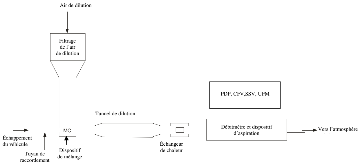
Figure A5/3 Système de dilution des gaz d'échappement
