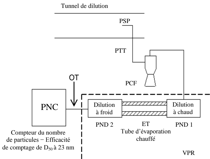
Figure A5/14 Système recommandé de prélèvement des particules
