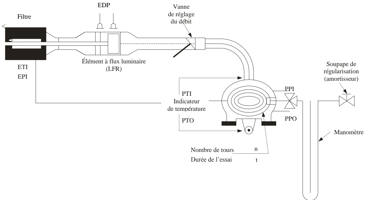
Figure A5/6 Configuration d'étalonnage pour système de prélèvement à pompe volumétrique
