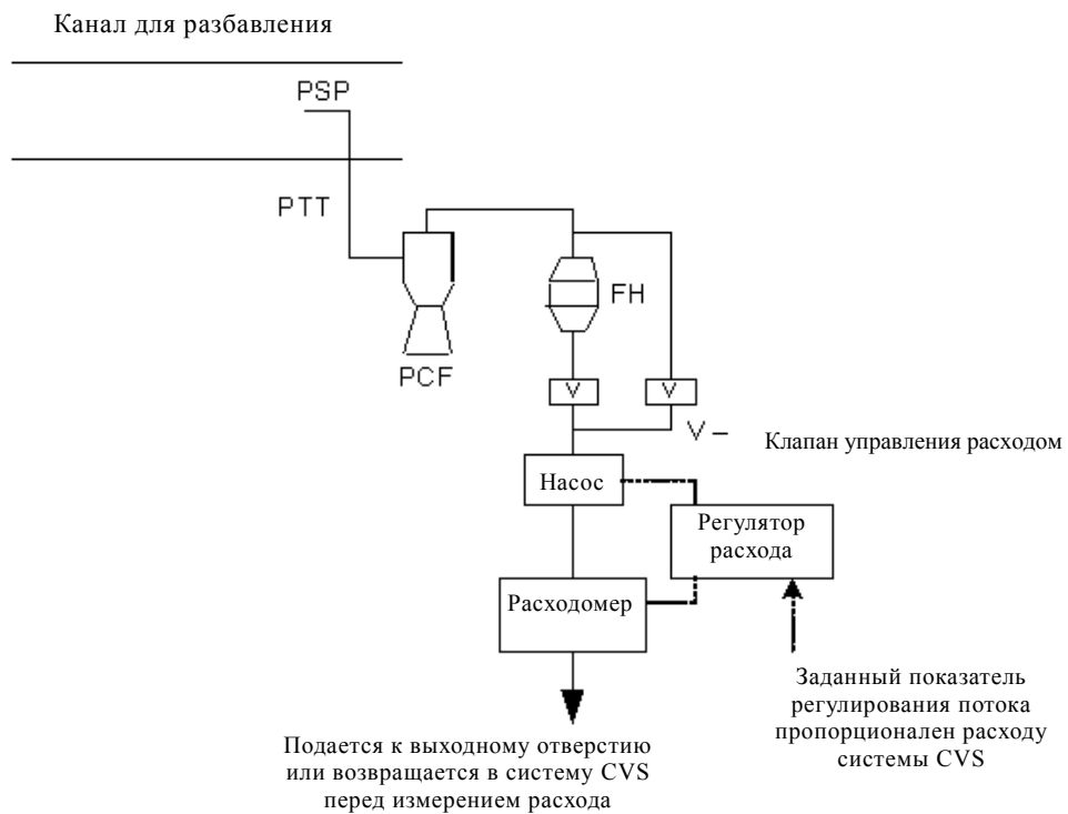
Рис. А5/12 Система отбора проб взвешенных частиц
