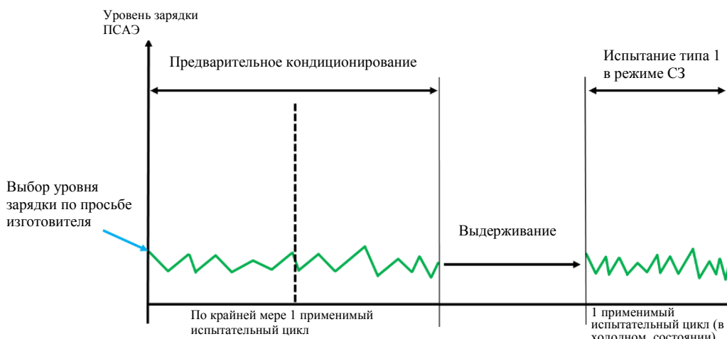
Рис. А8.App1/2 ГЭМ-ВЗУ, испытание типа 1 в режиме сохранения заряда
