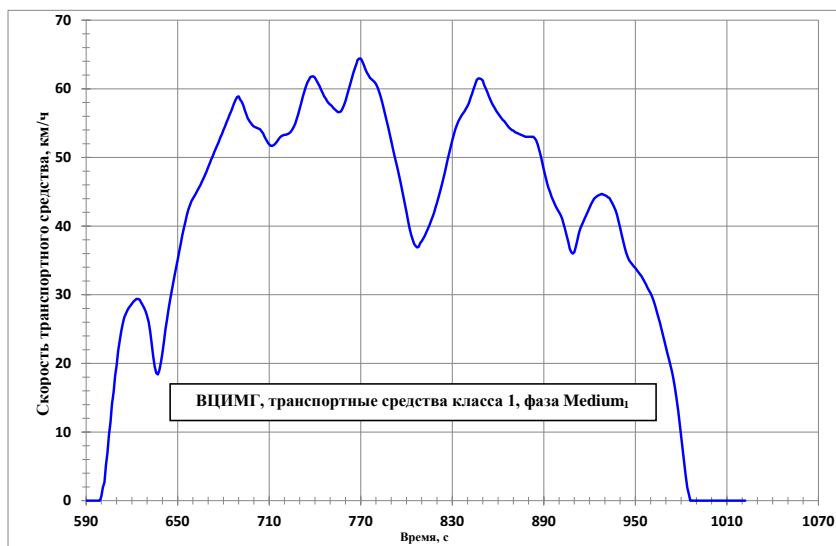
Рис. А1/2 ВЦИМГ, транспортные средства класса 1, фаза Medium 1
