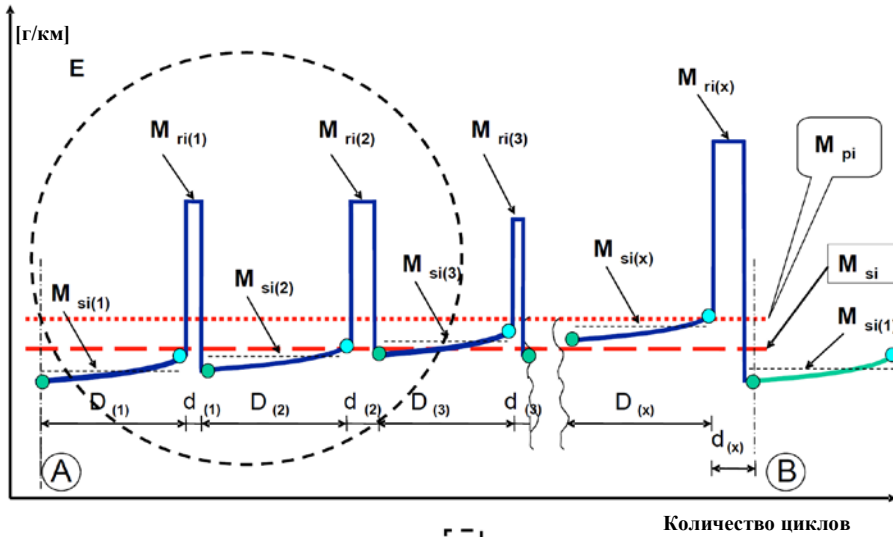
Рис. А6.Аpp1/2 Параметры, измеряемые в ходе испытания на выбросы во время циклов с регенерацией и между ними (условный пример)
