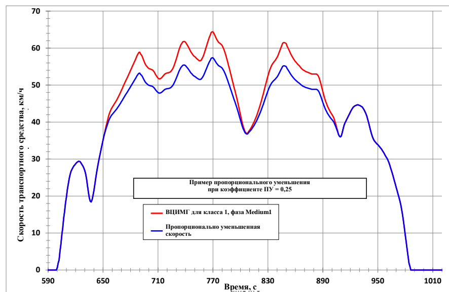
Рис. A1/13 Редуцированная фаза средней скорости ВЦИМГ для транспортных средств класса 1
