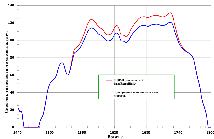
Рис. A1/15 Редуцированная фаза сверхвысокой скорости ВЦИМГ для транспортных средств класса 3
