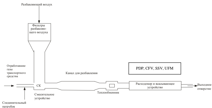
Рис. A5/3 Система разбавления отработавших газов
