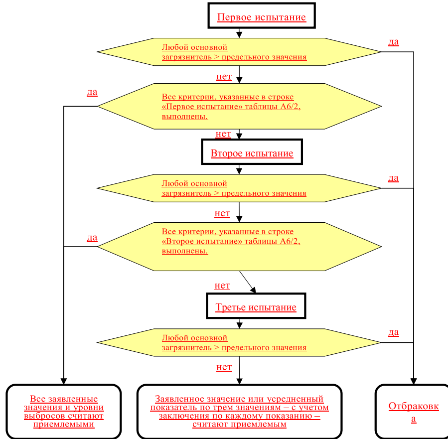
Рис. А6/1 Схема определения числа испытаний типа 1
