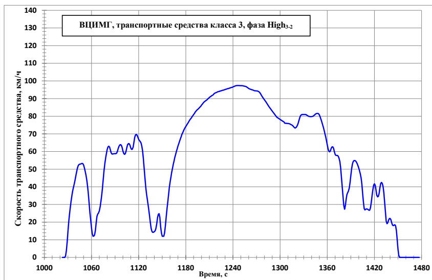
Рис. А1/11 ВЦИМГ, транспортные средства класса 3, фаза High 3,2
