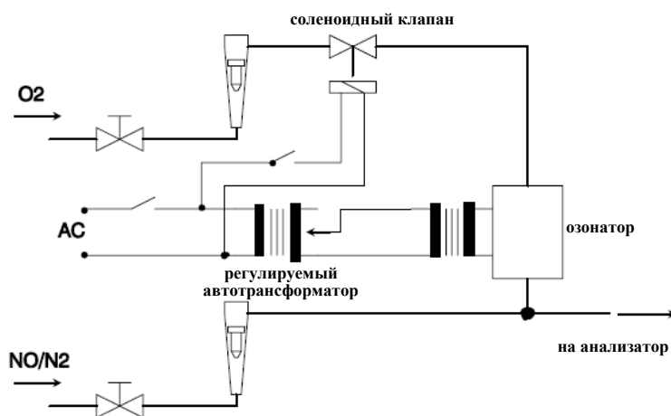
Схема испытания для проверки эффективности работы преобразователя \text{NO}_x
