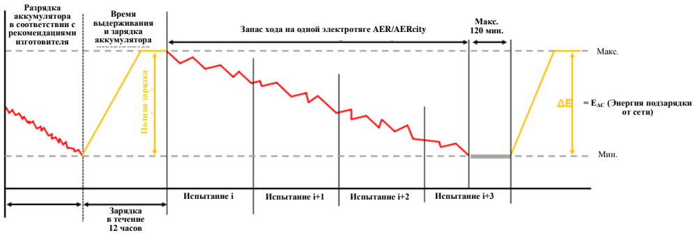
Рис. A8.App1e/1 Испытание ПЭМ для определения запаса хода на электротяге и расхода электрической энергии
