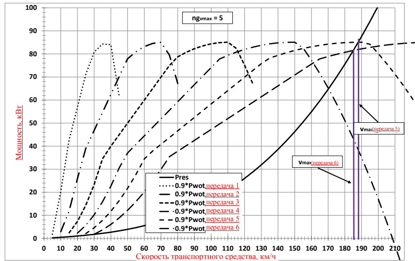
Рис. 1б Пример случая, когда ng_{vmax} является 2-й самой высокой передачей
