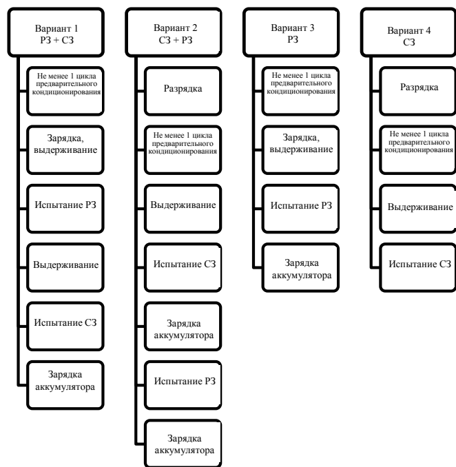
Рис. А8/1 Возможные варианты последовательности испытания ГЭМ-ВЗУ
