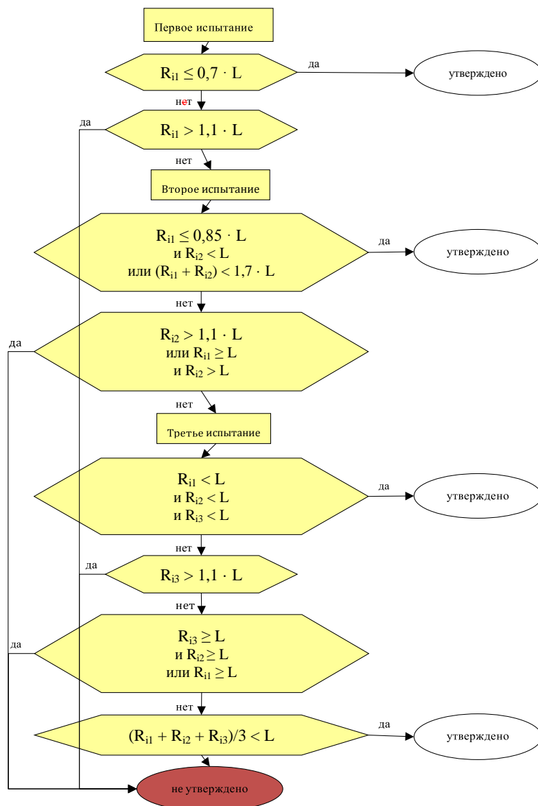
Рис. А6/4 Схема определения типа испытаний
