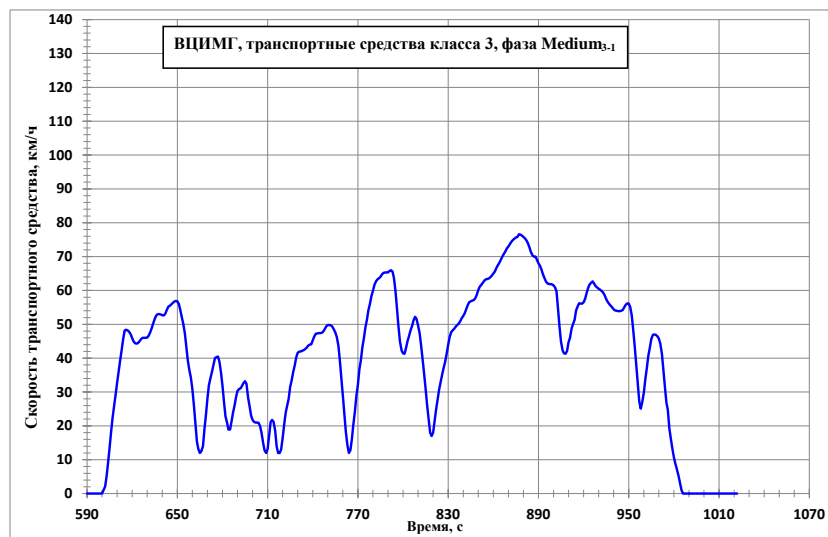
ВЦИМГ, транспортные средства класса 3, фаза Medium 3-1
