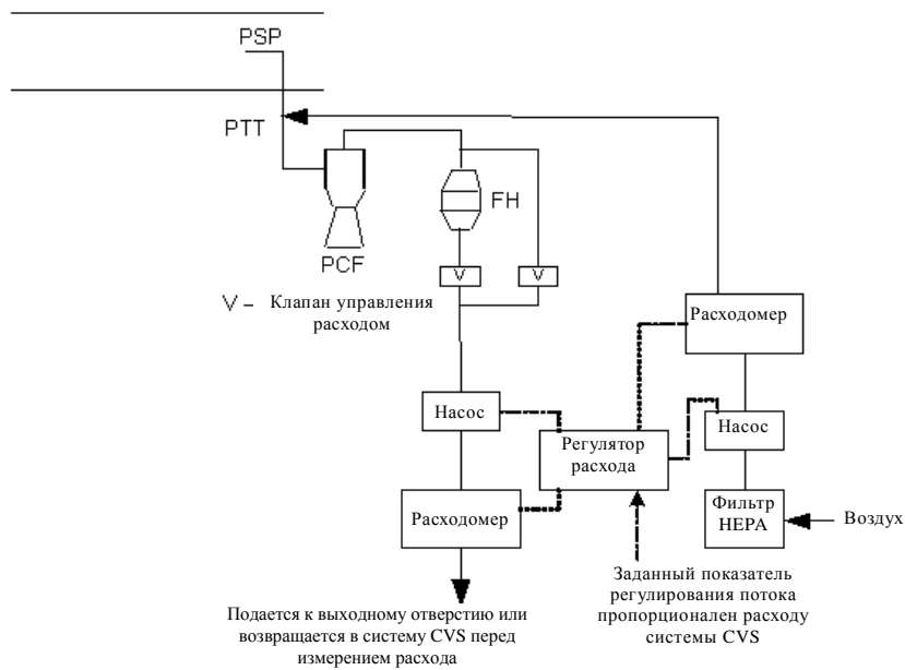
Рис. А5/ 42 13 Система отбора проб взвешенных частиц с двойным разбавлением
