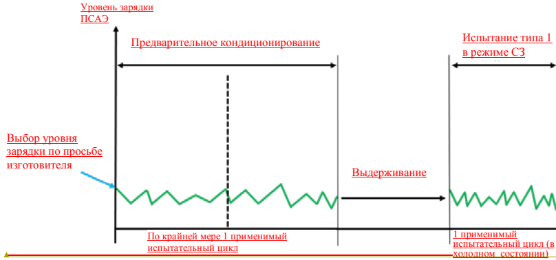
Рис. A8.App1/2 ГЭМ-ВЗУ, испытание типа 1 в режиме сохранения заряда
