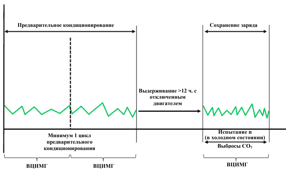
Рис. А8.Аpp1б/1 Испытание ГЭМ-ВЗУ в режиме сохранения заряда
