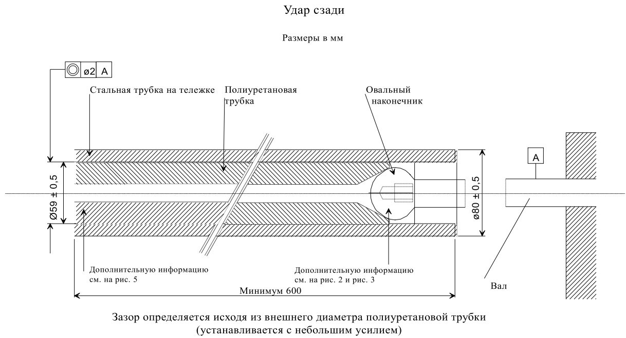
Рис. 4 Стопное устройство (в сборе)
