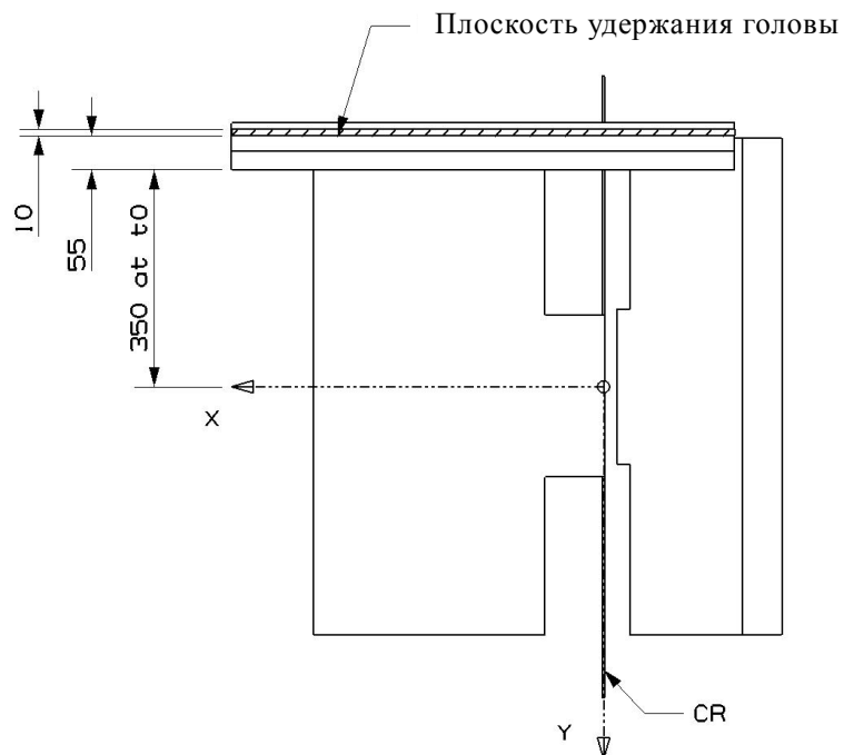
Рис. 1 Геометрия дверной панели и ее положение в момент T0 – Вид сверху
