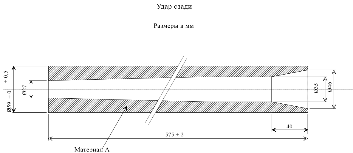
Рис. 5 Стопное устройство – полиуретановая трубка
