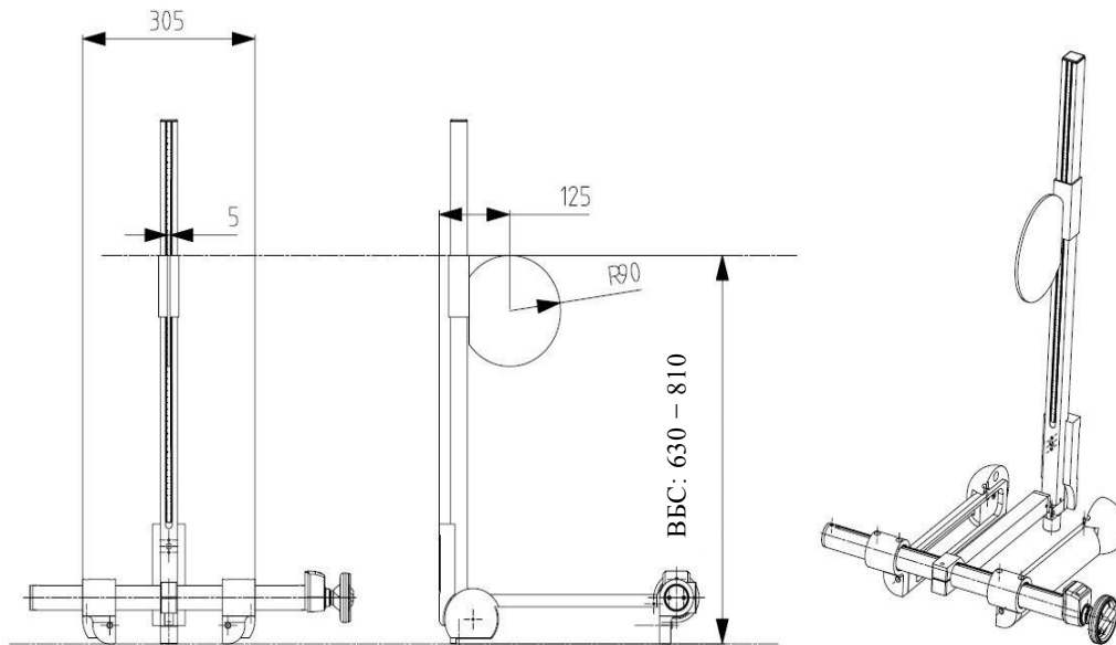
Рис. 1 Измерительное устройство для оценки универсальной бустерной подушки
