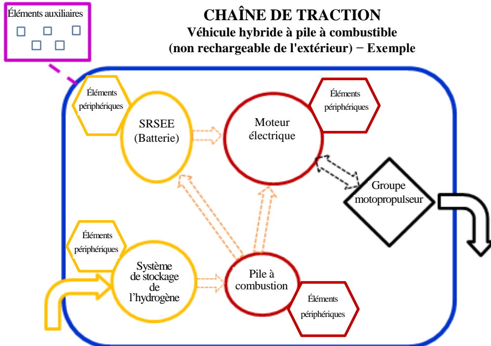
Figure 7 Véhicule hybride à pile à combustible (non rechargeable de l'extérieur)
