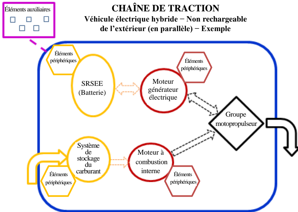
Figure 4 Véhicule électrique hybride – Non rechargeable de l'extérieur (en parallèle)
