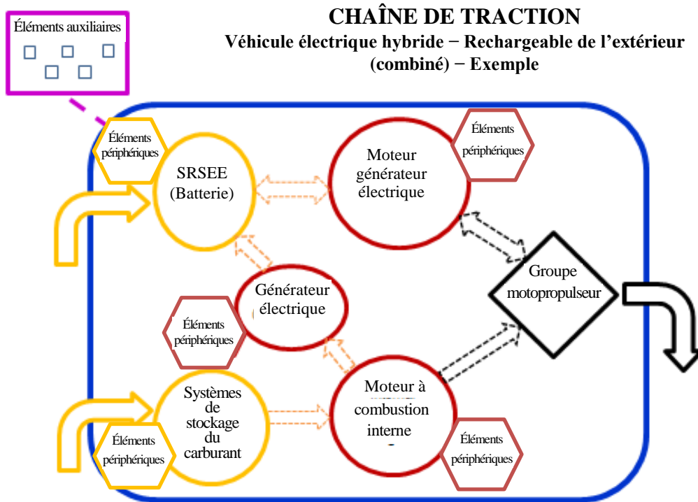
Figure 6 Véhicule électrique hybride – Rechargeable de l'extérieur (combiné)
