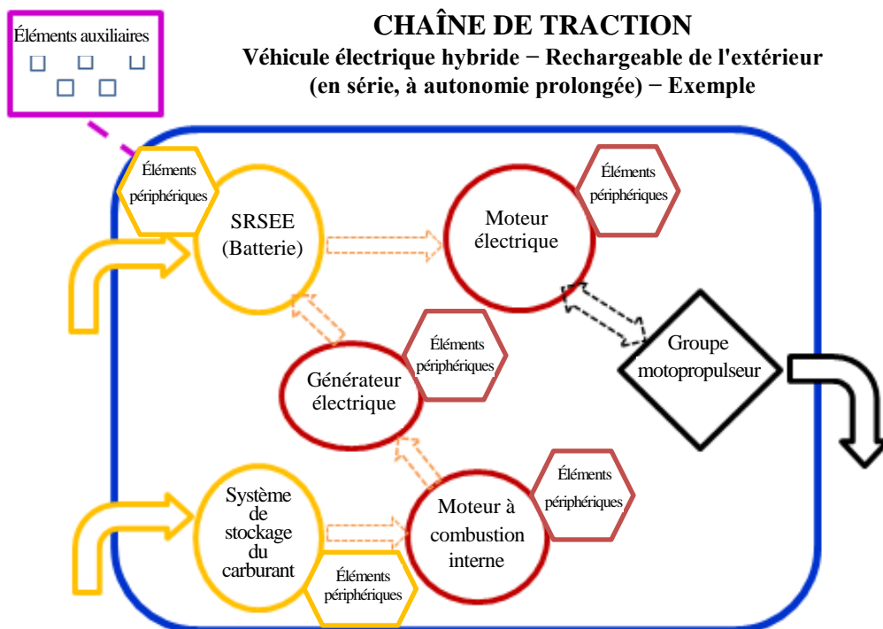
Figure 5 Véhicule électrique hybride – Rechargeable de l'extérieur (en série, à autonomie prolongée)
