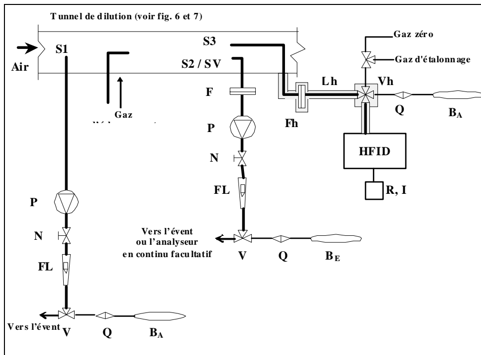
Figure A4a.App3/10 Schéma du système de prélèvement des émissions gazeuses
