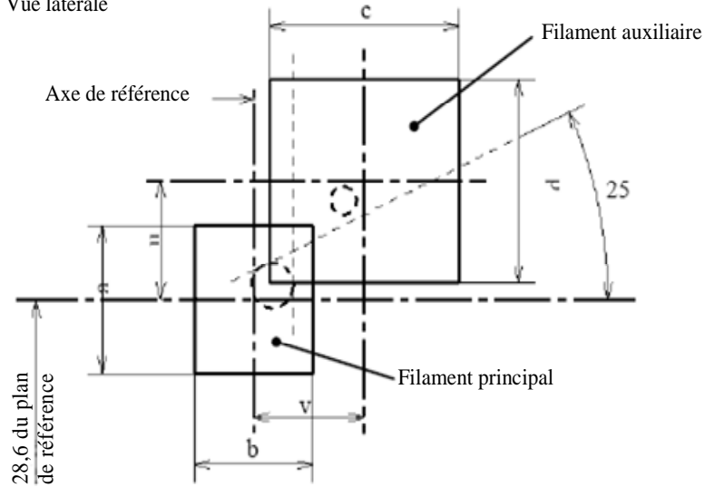
Vue latérale
