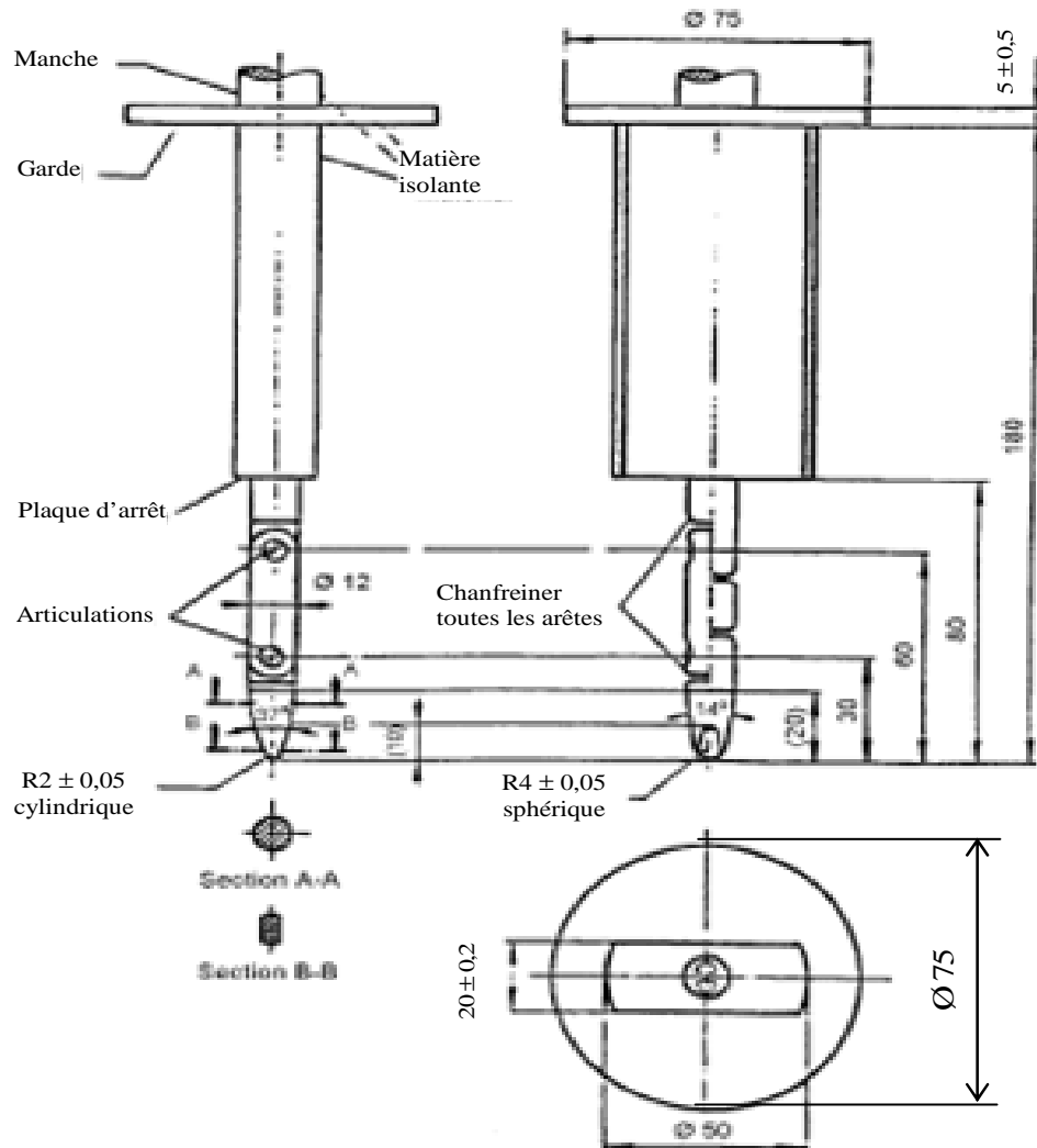
Figure 1 Doigt d'épreuve articulé
