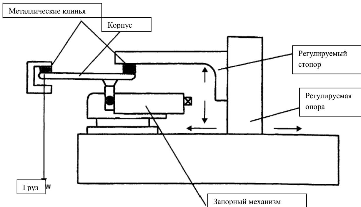
Рис. 2: Пример устройства испытания на изгиб для зеркала заднего вида
