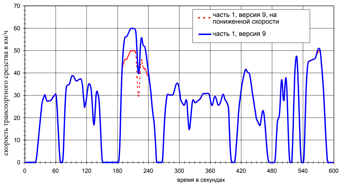
Диаграмма 11: Ездовой цикл ВЦИМ, часть 1
