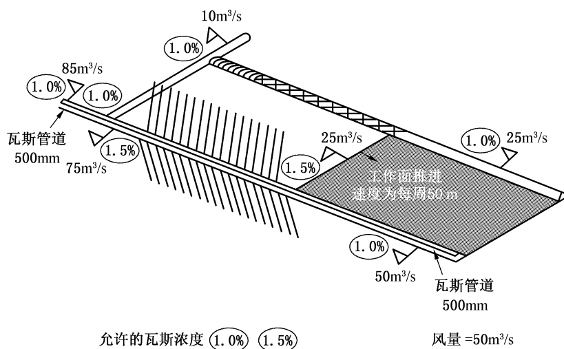
图 9-4 Y 型通风系统
