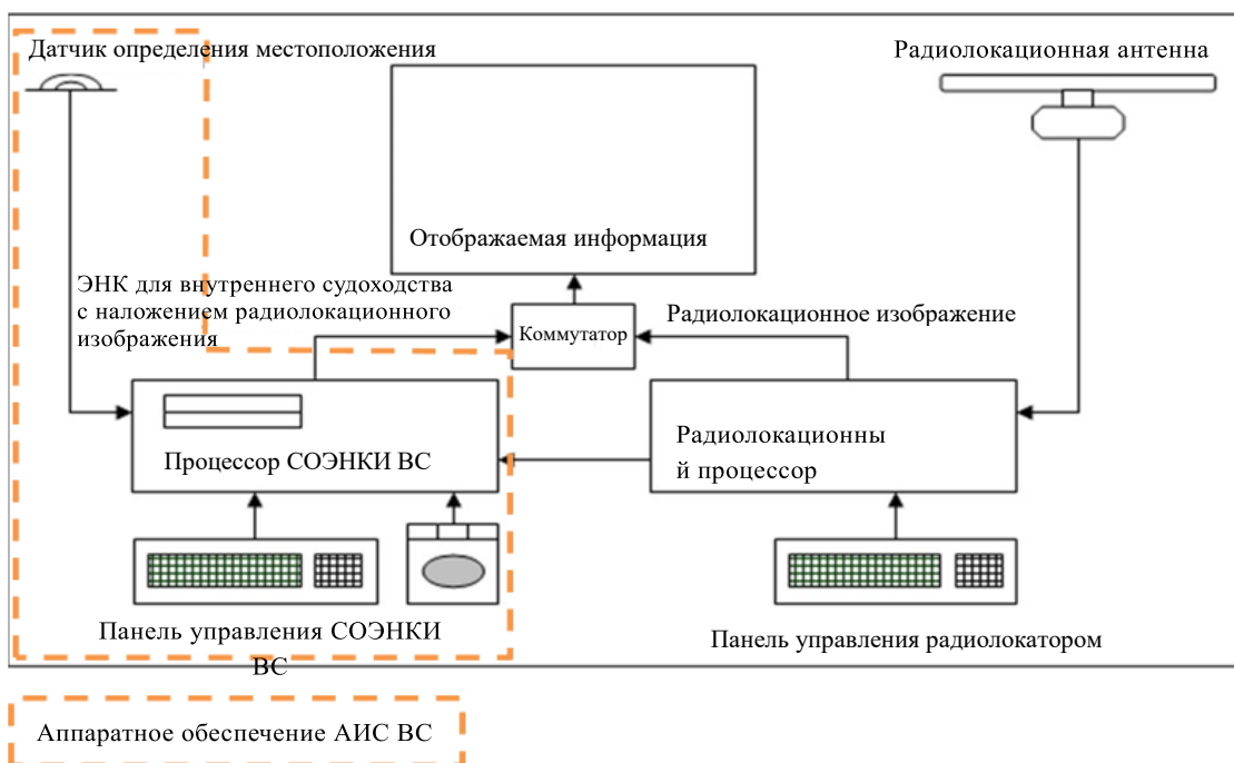
Рис. 2: Оборудование СОЭНКИ ВС, автономное оборудование, подсоединенное к радиолокационной станции и общему монитору (конфигурация системы 3)
