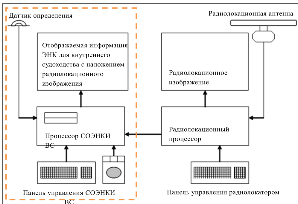
Рис. 2: Оборудование СОЭНКИ ВС, автономное оборудование, подсоединенное к радиолокационной станции и общему монитору (конфигурация системы 3)
