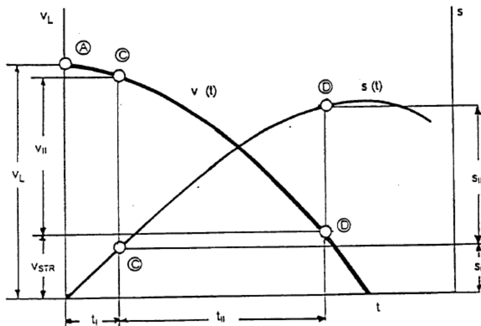
Рисунок 2: Расчет расстояния остановки
